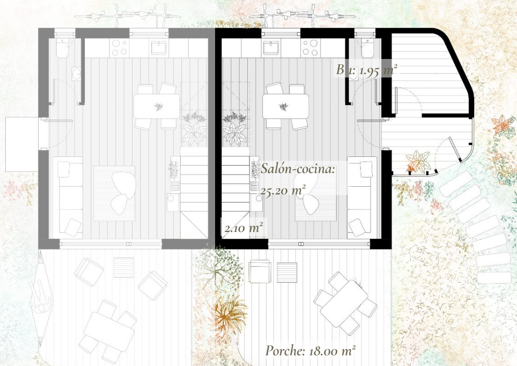
planta baja
